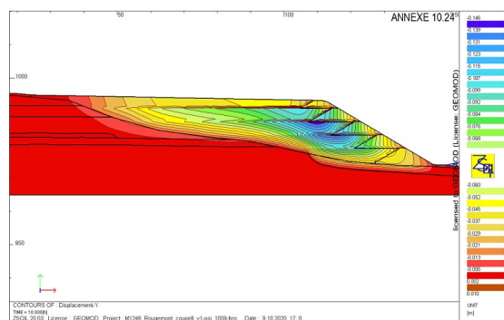
3.4a Résultats - Tassements - Etat final
